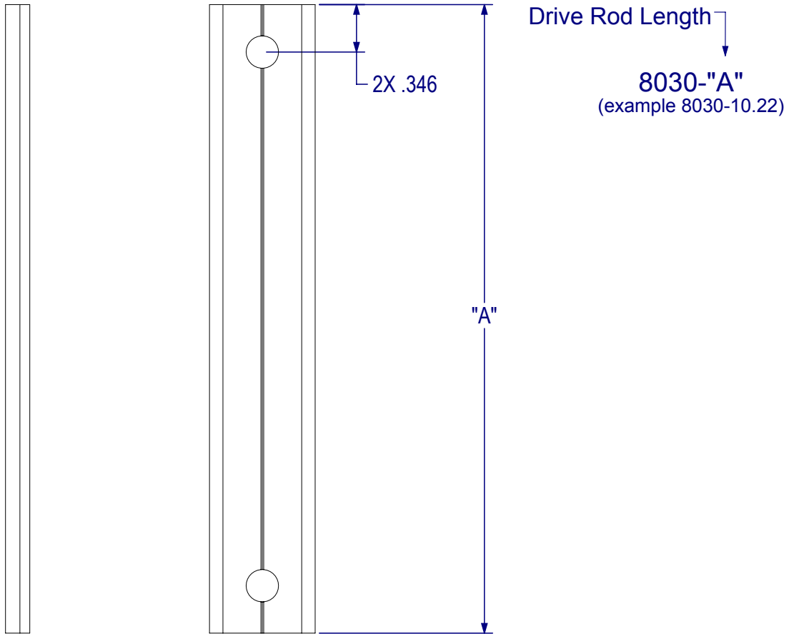
8030 Drive Rod
